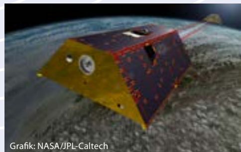
Grafik: NASA/JPL-Caltech
